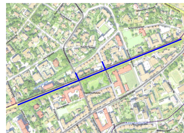
Sanierung Kanal (unterirdisch - grabenarm)
